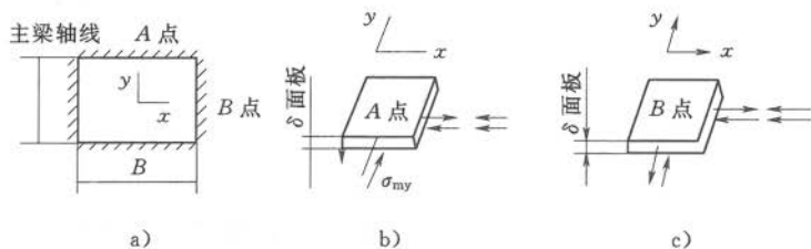
a) 面板计算区格；b) 支承长边中点 (A 点) 应力情况； c) 支承短边中点 (B 点) 应力情况
