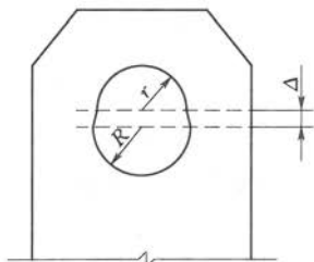
图 7.3.7 吊耳梨形孔
