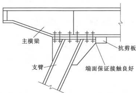
图 6.1.12 支臂抗剪板
