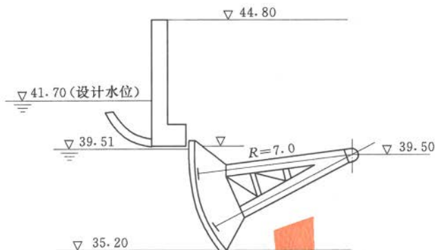
图1 鹤地水库弧形闸门的布置简图
